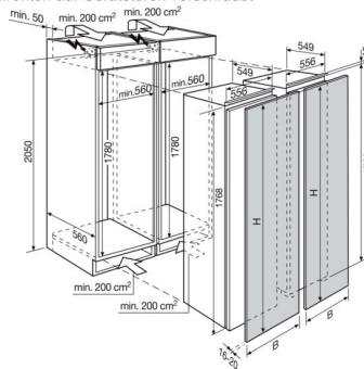
IK3035SZ und IG2085SN – Euro-Einbau Möbelfronten auf Gerätetüren verschraubt
