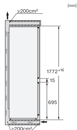
KFN7795D, Seitenansicht (Skizze)
