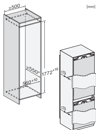
KFN7795D, Einbau (Fußnote*) (Skizze)
