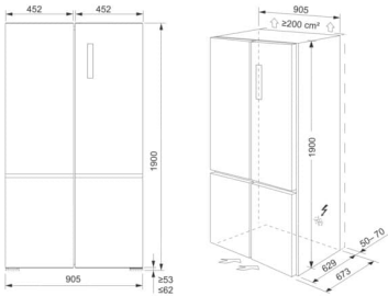
MD530NOCN (ohne Wasseranschluss)
