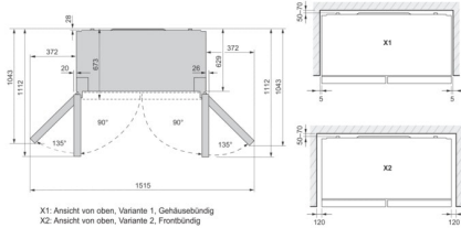
MD530NOCN (Ansicht von oben)
