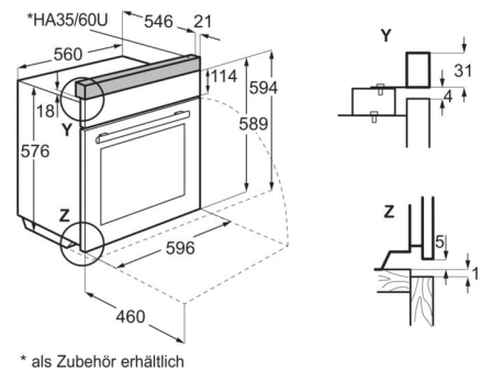
Einbaubackofen/Einbauherd + Höhenadapter EB6.../EH6... + HA35/60U
