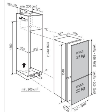
IK279BN / IK277BN / IK275BN Möbelfronten auf Gerätetüren verschraubt
