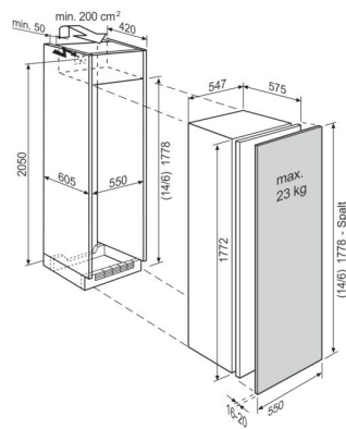
IK329SA / IK327SA
