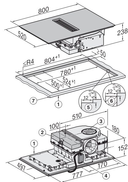
Tischlüfter TwoInOne KMDA 7876 FL-A, flächenbündig
