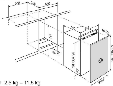
GA55SLV/GLV/LV + GAES55/35
