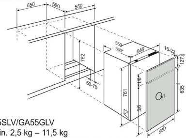
GA55SLV/GLV/LV
