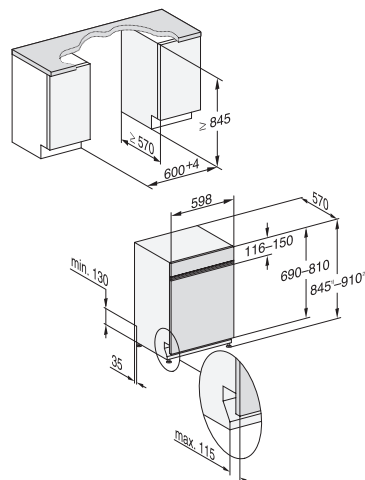
G 2xxxx-60 i, integrierbar
