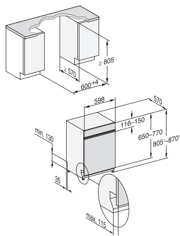
G 1xxxx-60 i, integrierbar
