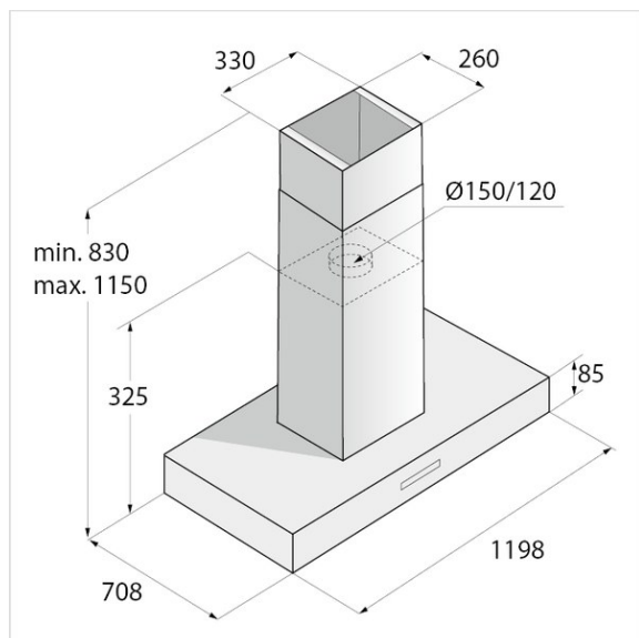
CI41230G Skizze
