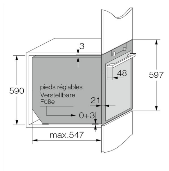
OP8687B 2 Skizze
