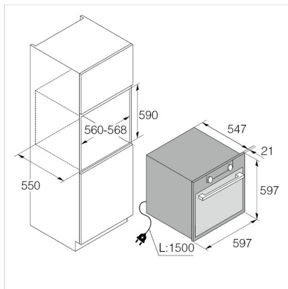
OP8687B 1 Skizze
