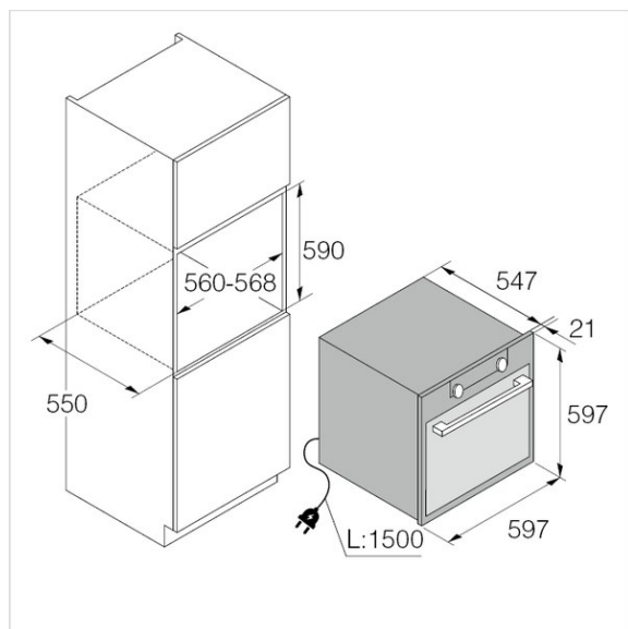
OP8687A 1 Skizze
